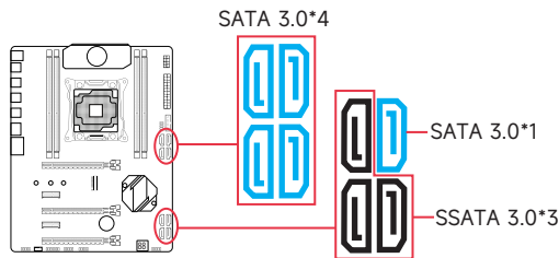
图2 -10 SATA接口
