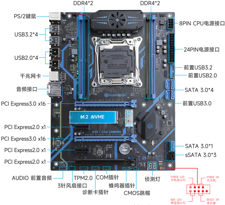
图1-1 X99-CD4 GAMING主板图解
